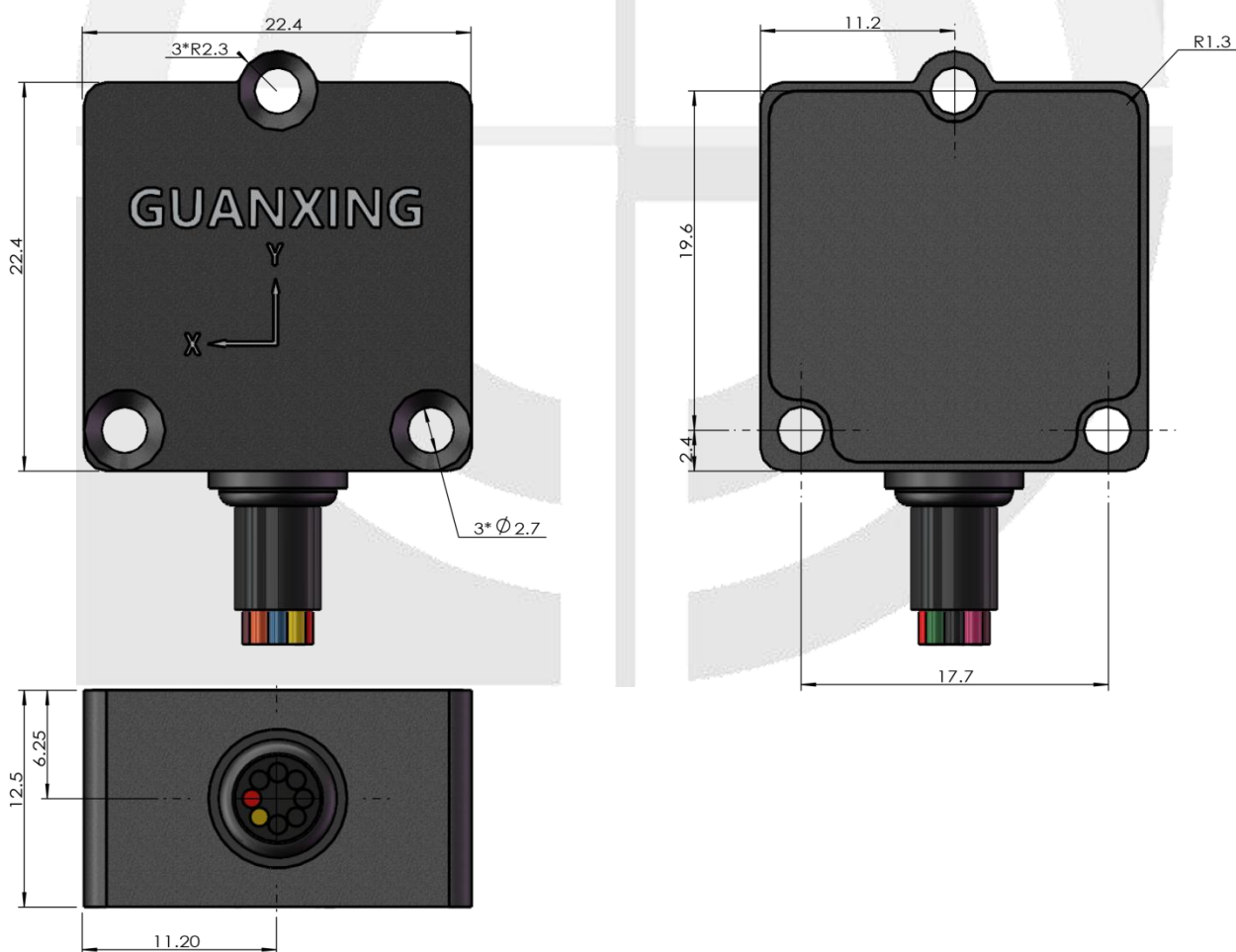
图 7 传感器主体各部位尺寸
