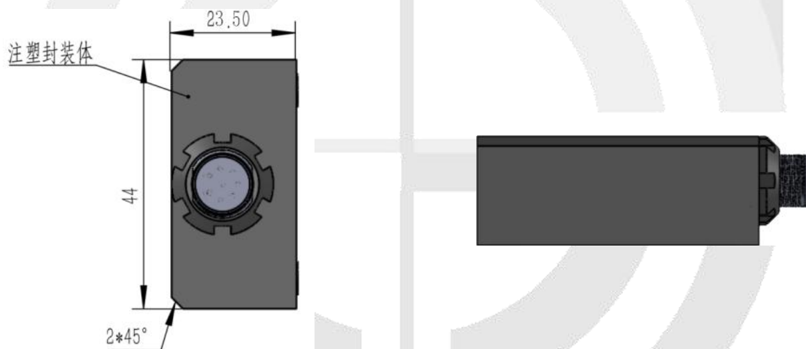
图 7 传感器主体各部位尺寸
