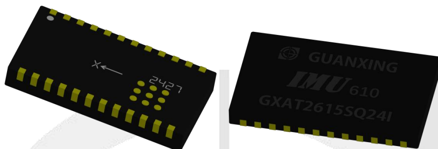
图 9 运动姿态传感器微系统芯片 IMUi610/611 外形图
