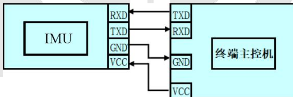
图6 串口传输示意图
