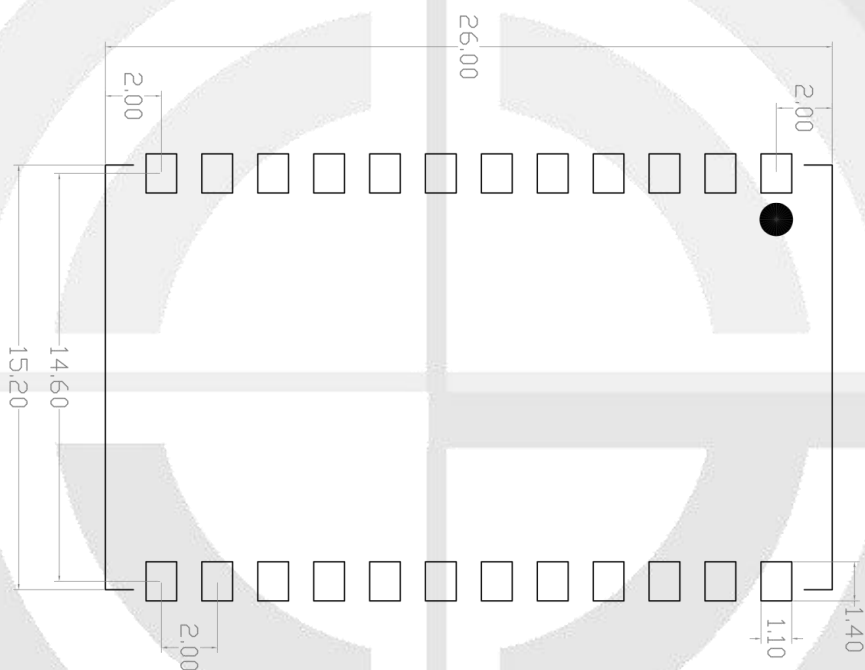
图11 运动姿态传感器微系统芯片 IMU610推荐 PCB 焊盘布局
