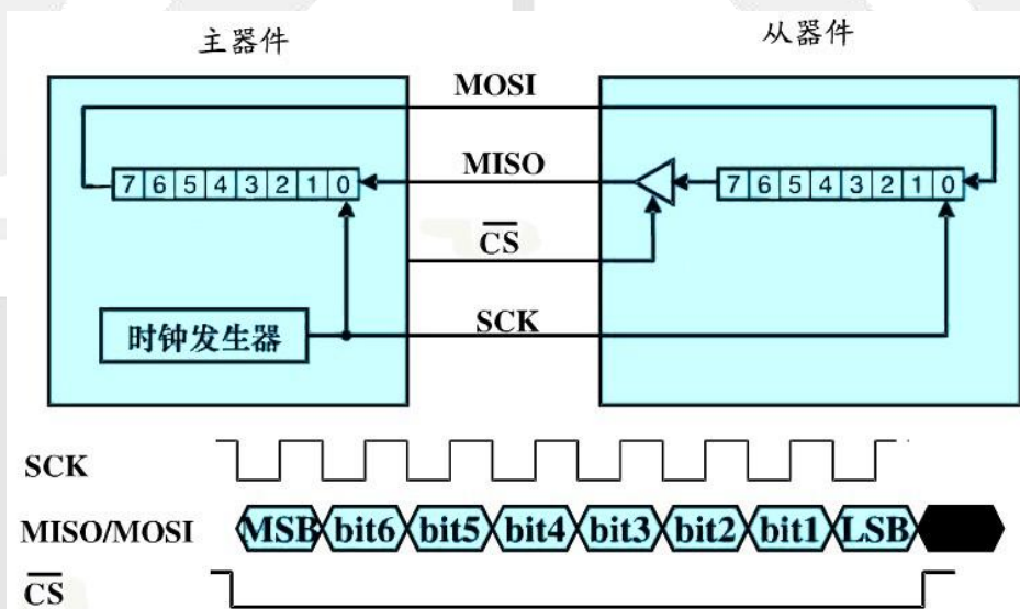
图 7 SPI 传输示意图
