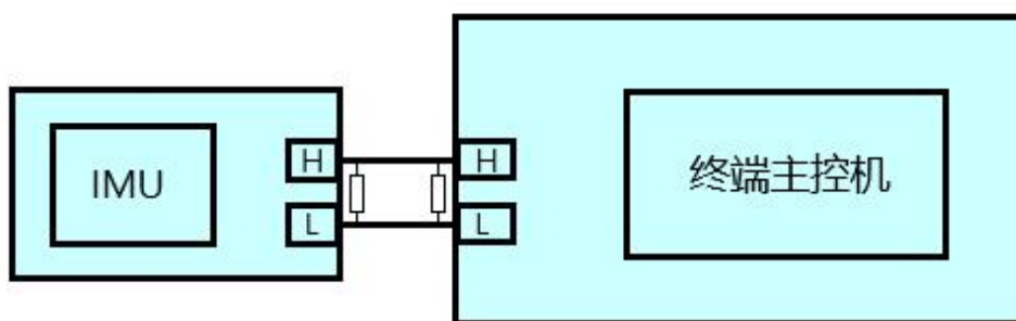
图8 CAN 传输示意图
