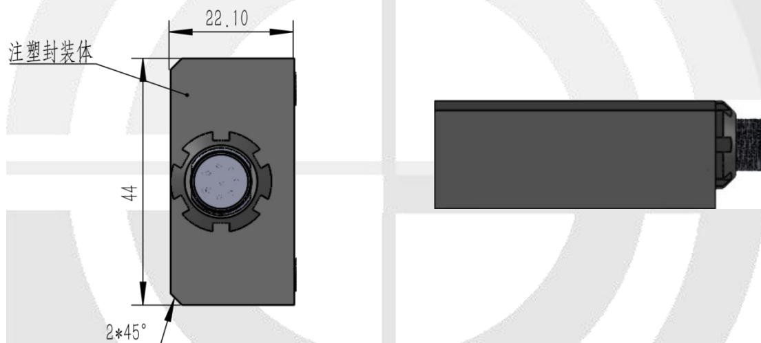
图 7 传感器主体各部位尺寸
