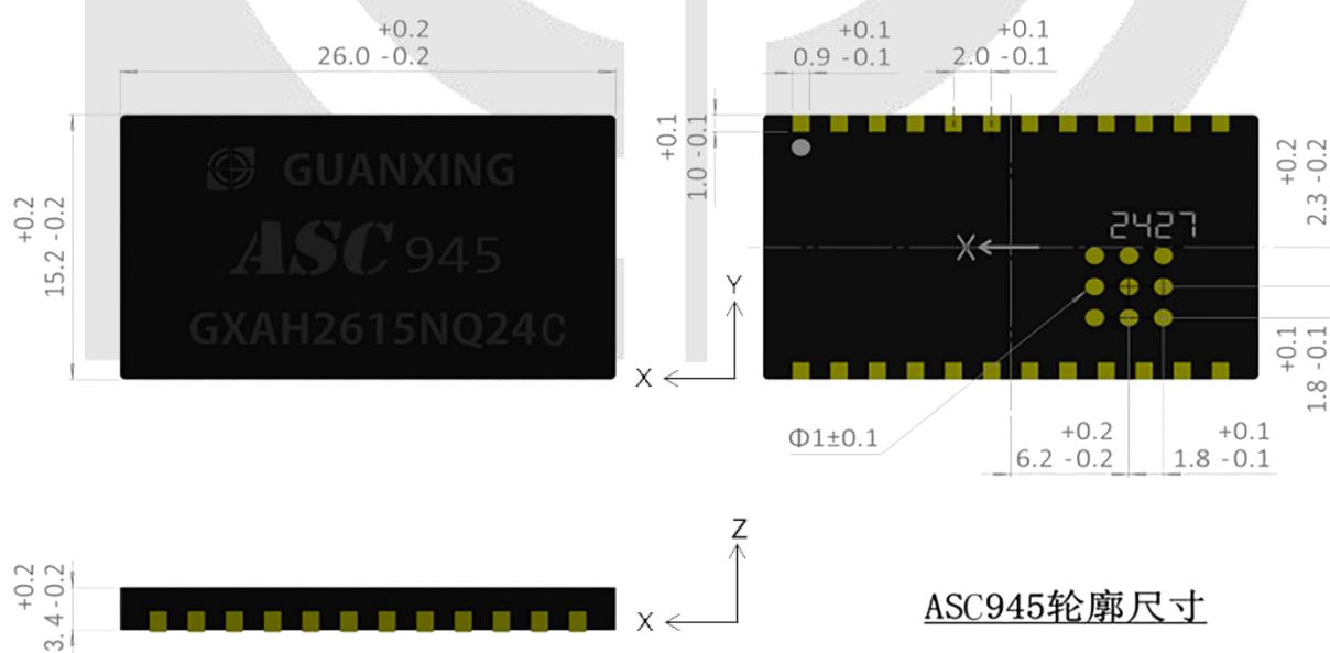
图10 姿态航向传感器微系统芯片 ASC945封装尺寸
