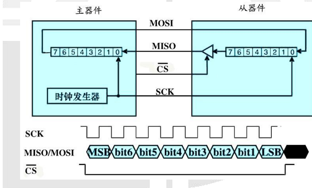
图 7 SPI 传输示意图
