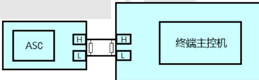
图8 CAN 传输示意图
