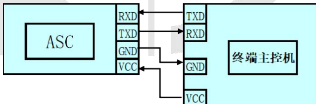
图6 串口传输示意图
