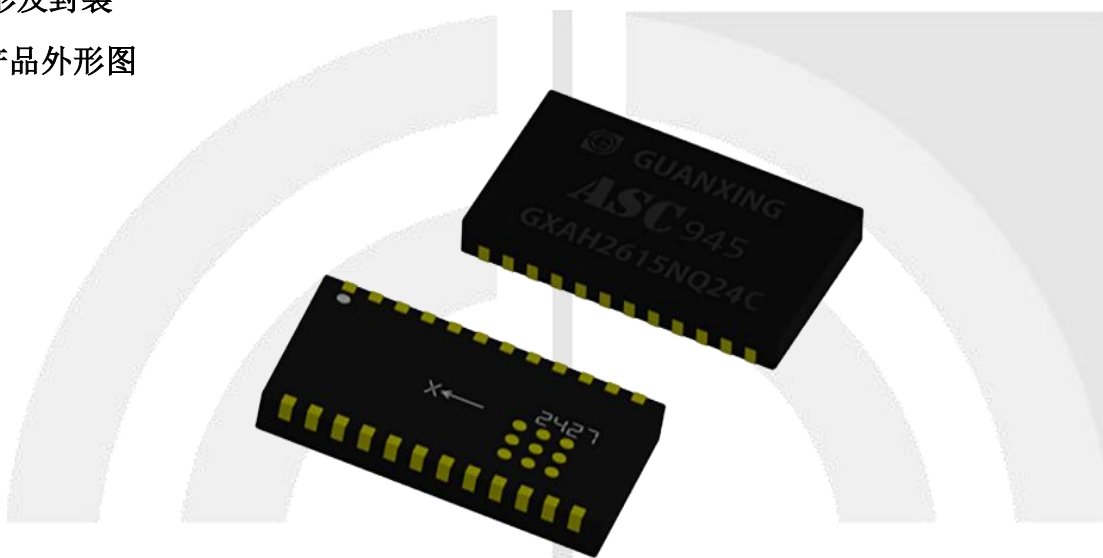
图9 姿态航向传感器微系统芯片 ASC945 外形图
