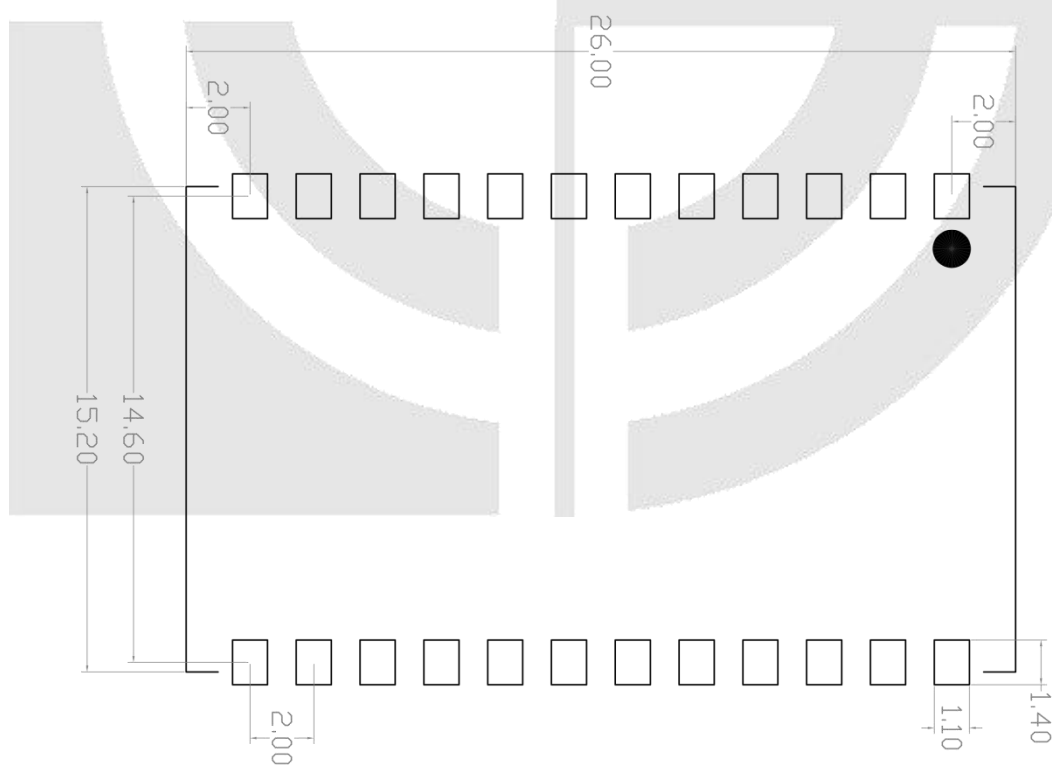
图11 运动姿态传感器微系统芯片 IMUi610/611推荐 PCB 焊盘布局
