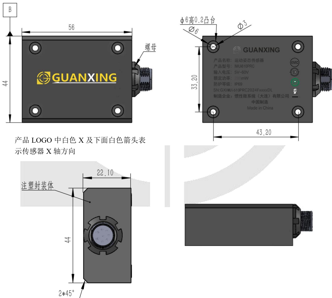
图 7 传感器主体各部位尺寸
