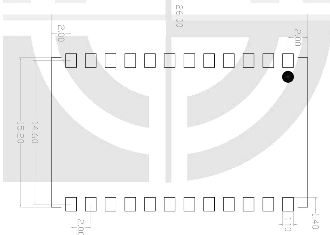
图 11 倾角传感器微系统芯片 VRU620 推荐 PCB 焊盘布局
