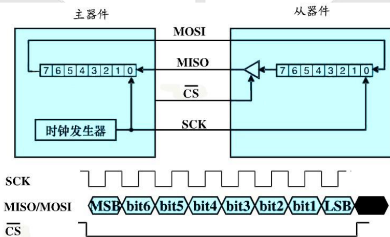
图7 SPI 传输示意图
