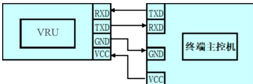
图6 串口传输示意图
