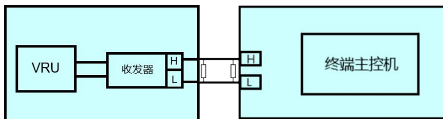
图8 CAN 传输示意图
