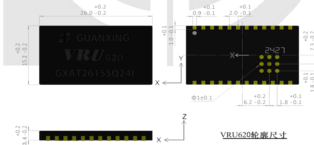
图10 倾角传感器微系统芯片 VRU620封装尺寸
