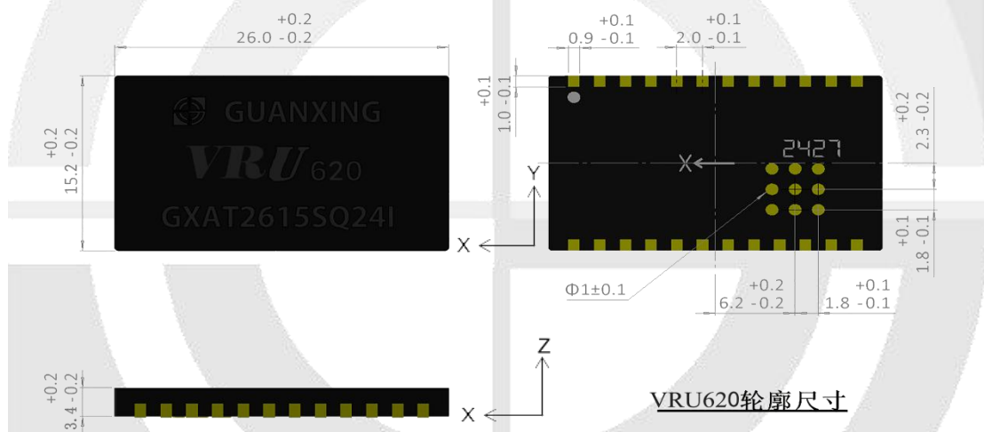
图9 倾角传感器微系统芯片 VRU620封装尺寸与轴向
