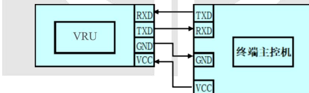
图5 串口传输示意图
