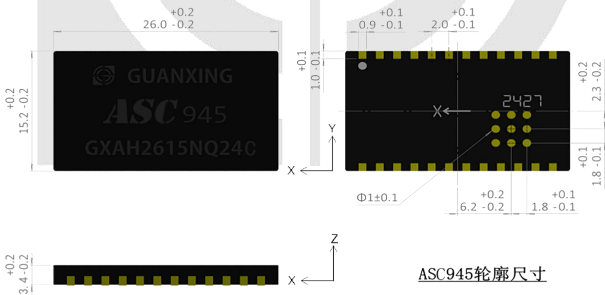
图11 姿态航向传感器微系统芯片 ASC945封装尺寸与轴向
