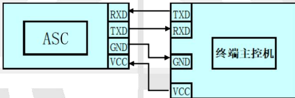
图7 串口传输示意图
