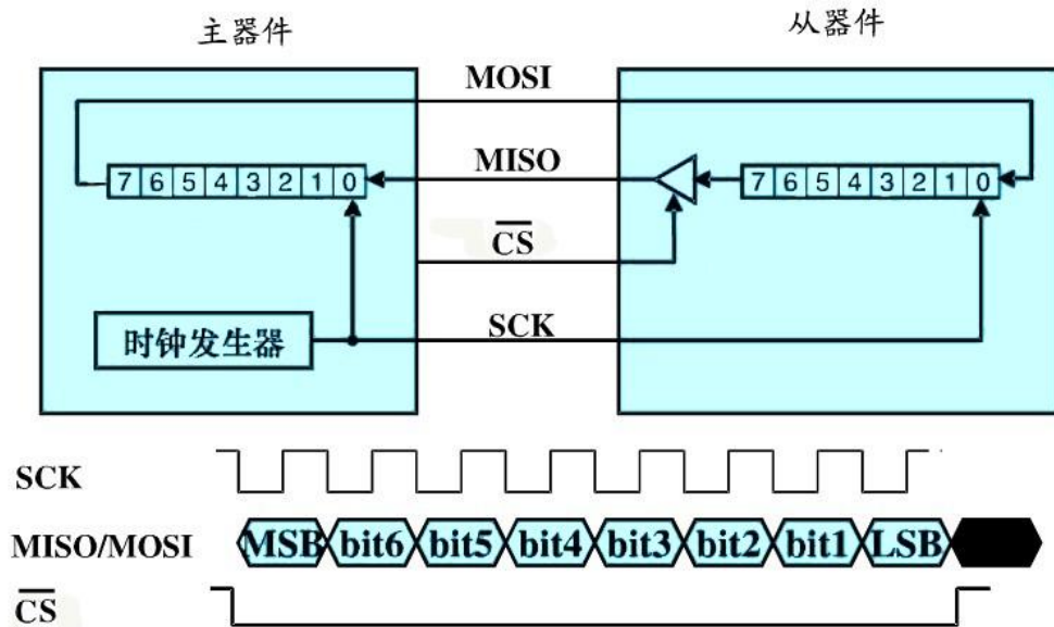
图 8 SPI 传输示意图
