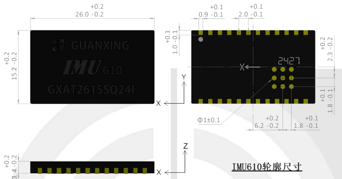
图9 运动姿态传感器微系统芯片 IMU610封装尺寸与轴向
