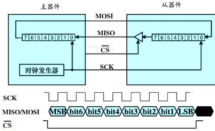
图 6 SPI 传输示意图
