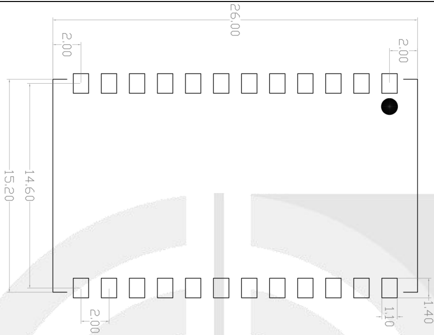
图10 运动姿态传感器微系统芯片 IMU610推荐 PCB 焊盘布局
