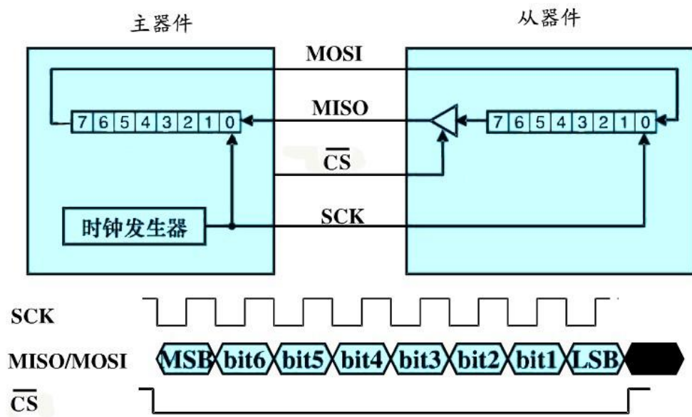
图 6 SPI 传输协议
