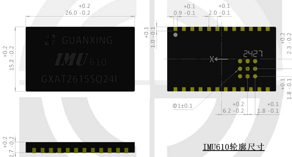
图9 运动姿态传感器微系统芯片封装尺寸
