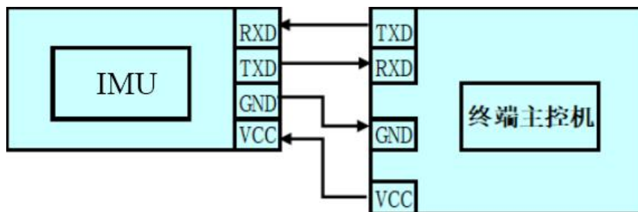
图5 传感器与终端主控机连接示意图
