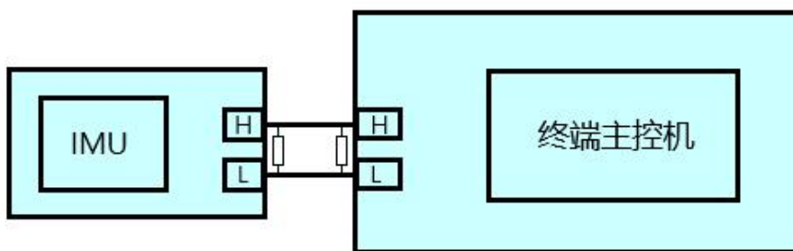
图7 IMU 与终端主控机 CAN 连接示意图
